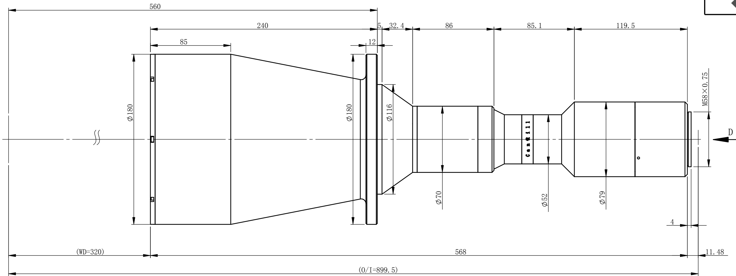
视图 D 1 : 2.5
