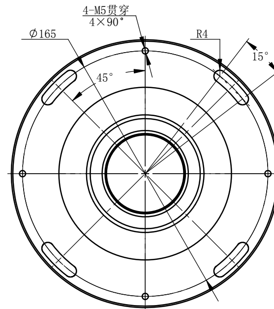
视图 D 1 : 2.5
