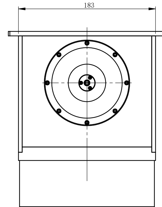
视图G
